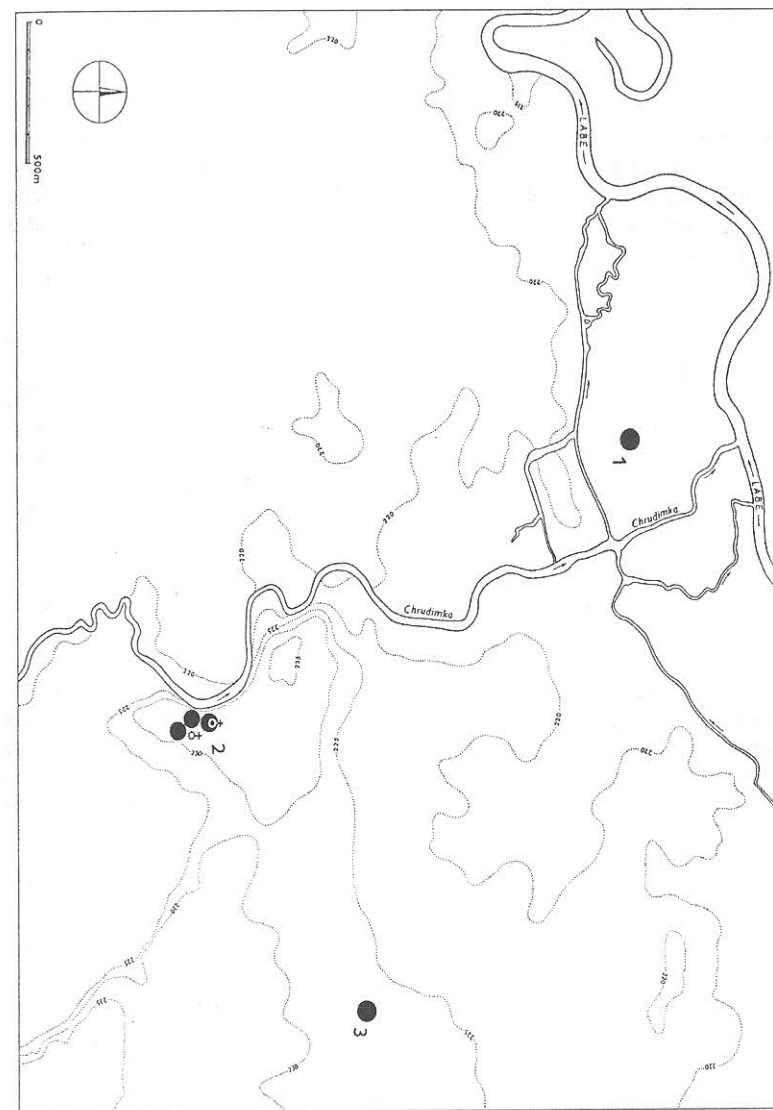
Obr.: Terénní reliéf dnešních Pardubic (vodní toky podle stabilního katastru z r. 1839). Zakresleny známé polohy kostelů ze 13. století (kostel sv. Jiljí a kostel v zaniklém církevním komplexu) a vyznačena místa s archeologickými doklady osídlení ve 13. století: 1 - zámek, 2 - Pardubičky, 3 - Slovaný. Kreslila M. Záleská.
